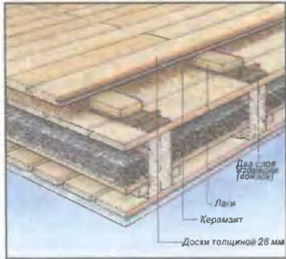
Рис. 2. Вариант звукоизоляции пола. Старое перекрытие не меняют на новое. Его застилают плотной бумагой, препятствующей попаданию в щели засыпки. На полосы звукоизоляции (войлок или строительный картон) кладут лаги (6х6 см). К ним крепят доски нового покрытия пола. Чтобы пол не скрипел, можно укладывать новое
